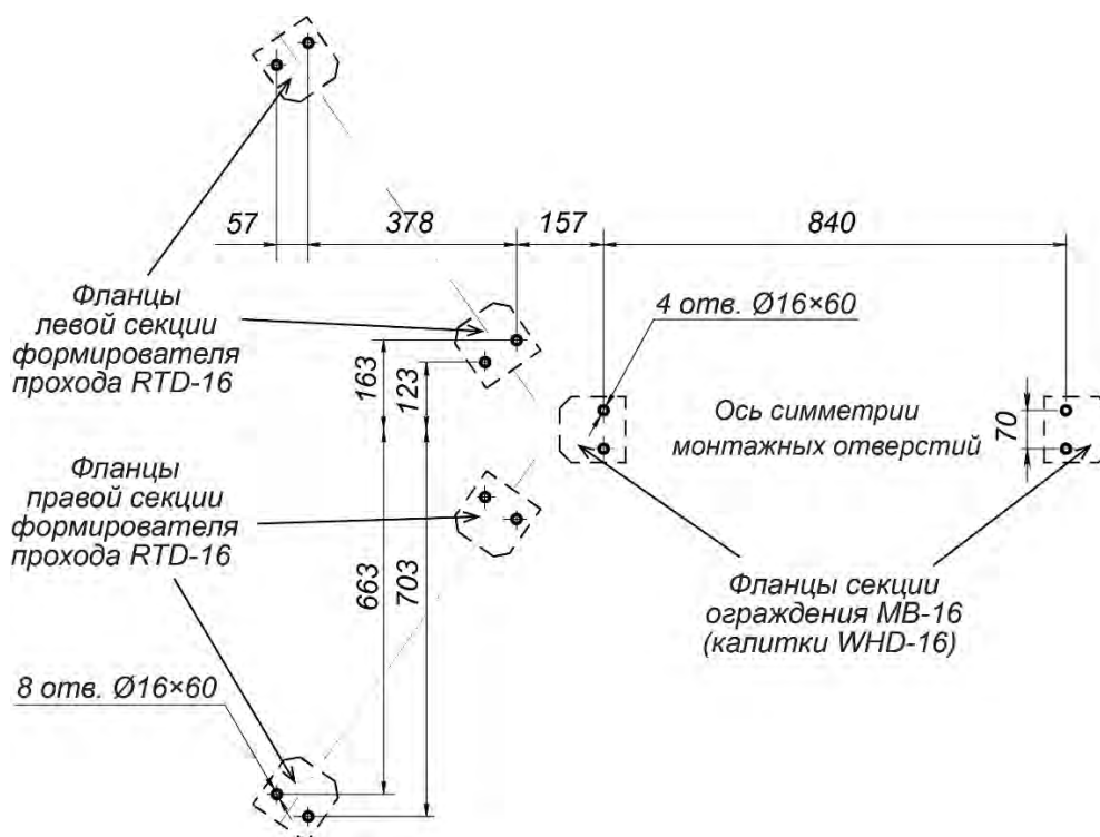
Рисунок 28. Схема разметки для монтажа турникета с ограждением или калиткой, расположенными со стороны секций формирователя прохода..
