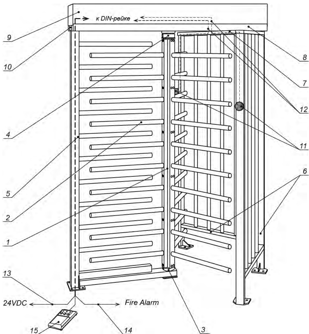
Рисунок 2. Устройство турникета:
