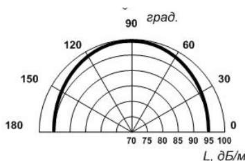
Рисунок 1 – Диаграмма направленности оповещателя
