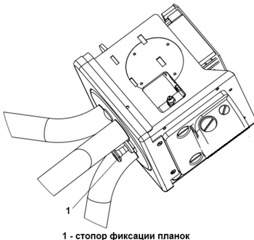
Рисунок 6 – Стопор фиксации планок
