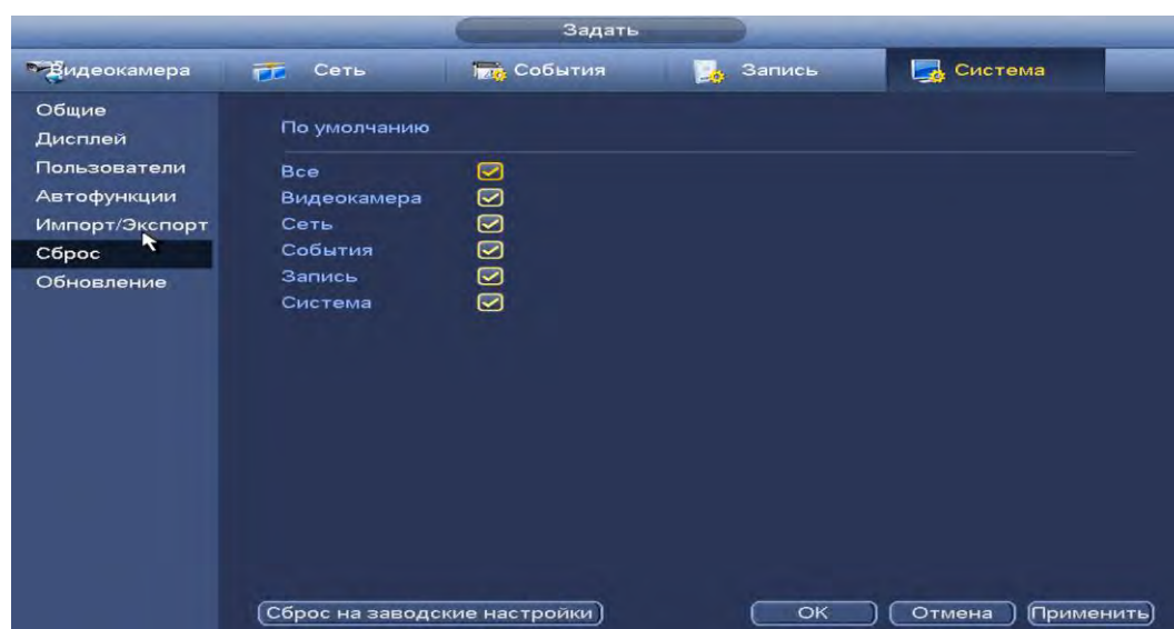
Рисунок 8.135 Интерфейс настройки сброса.
