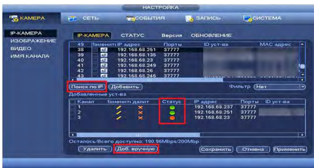
Рисунок 8.30 Интерфейс добавления камер к устройству.
