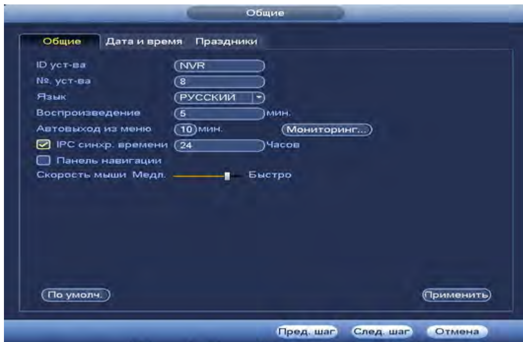
Рисунок 6.5 Интерфейс меню быстрой настройки «Общие».
