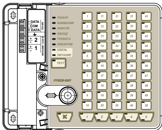
Рисунок 1 - Внешний вид прибора
