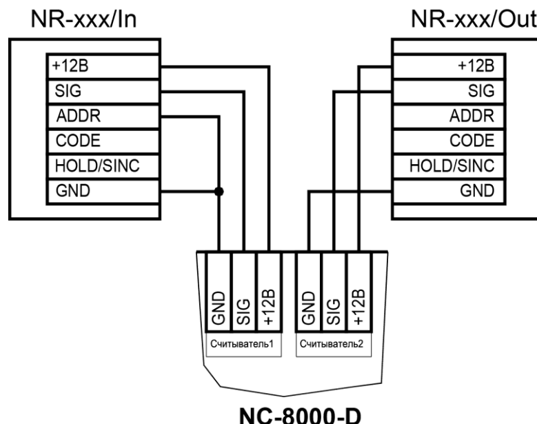
Рисунок 7. Схема подключения считывателей серии NR к контроллеру двумя кабелями
