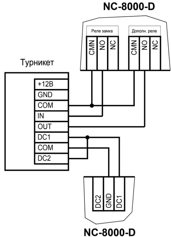
Рисунок 11. Схема подключения контроллера к турникету
