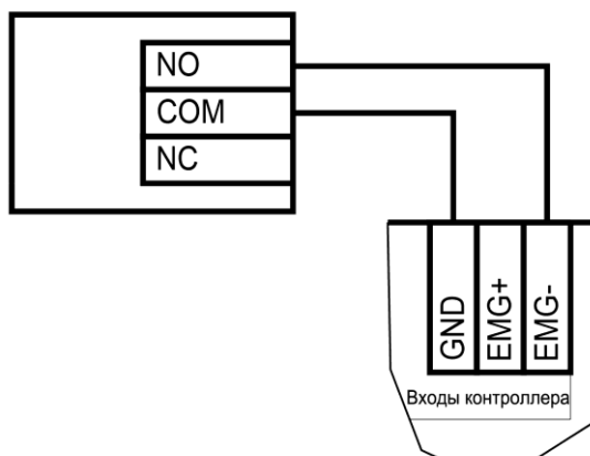
Рисунок 18. Схема подключения кнопки аварийного выхода к одному контроллеру
