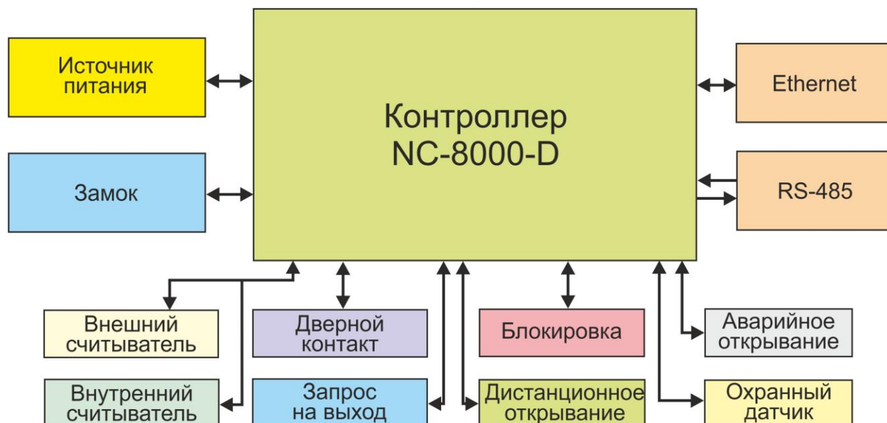
Рисунок 5. Оборудование, подключаемое к контроллеру NC-8000-D
