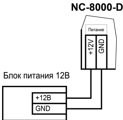
Рисунок 4. Схема подключения источника питания
