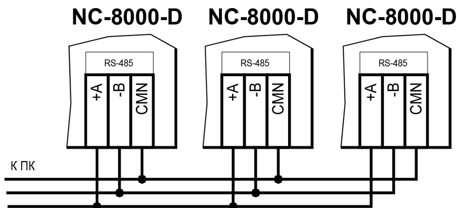
Рисунок 20. Схема соединения контроллеров по топологии «Шина»
