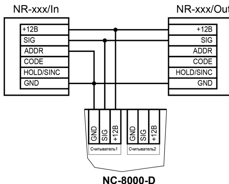
Рисунок 6. Схема подключения считывателей серии NR к контроллеру одним кабелем
