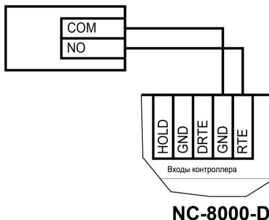
Рисунок 12. Схема подключения кнопки запроса на выход
