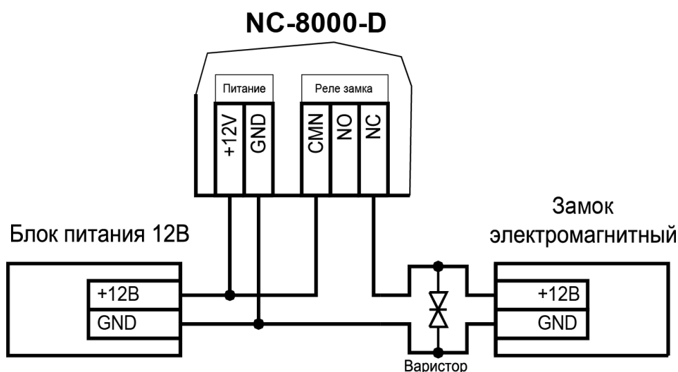
Рисунок 10. Схема подключения замка при питании от того же источника, что и контроллер
