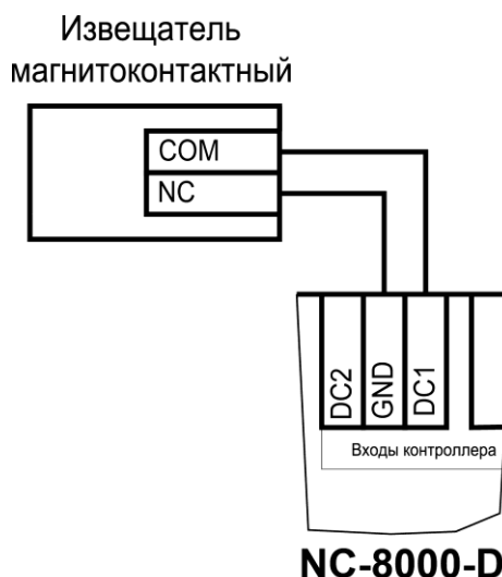
Рисунок 14. Схема подключения дверного контакта
