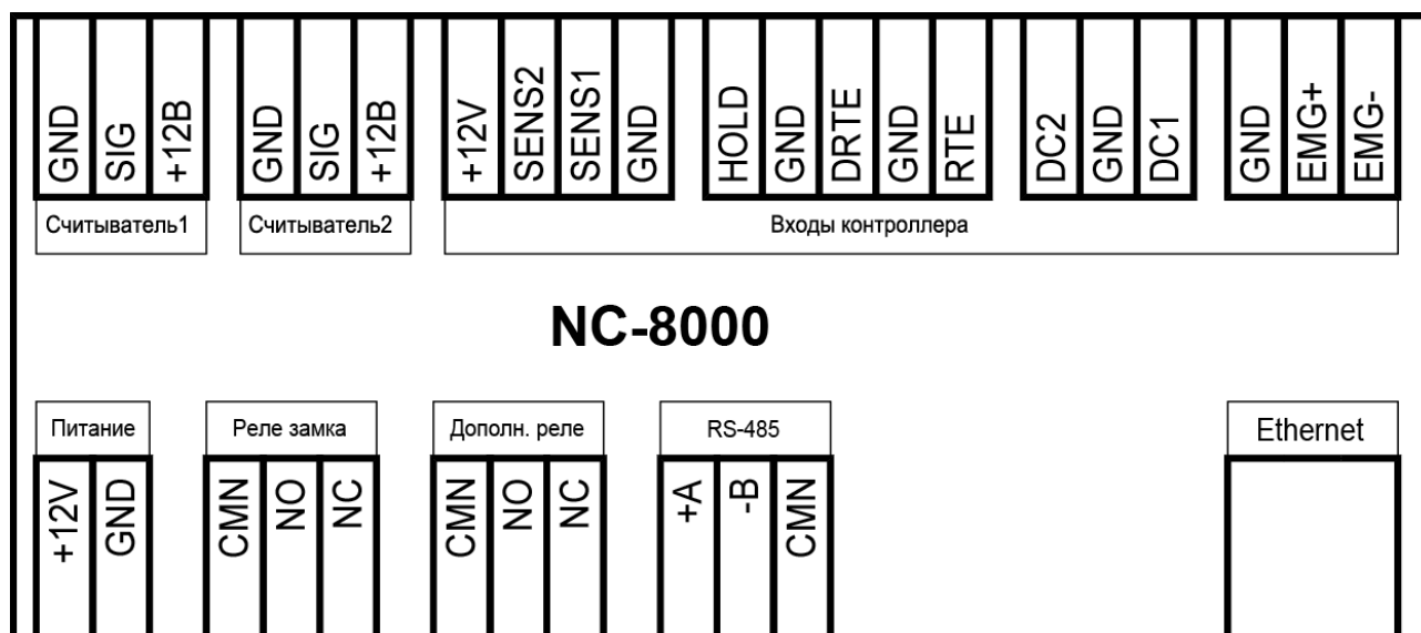
Рисунок 2. Маркировка клемм на крышке контроллера
