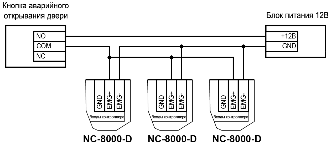
Рисунок 19. Схема подключения одной аварийной кнопки к нескольким контроллерам
