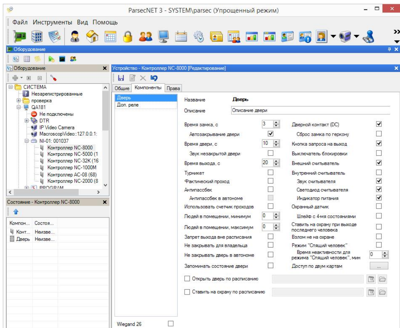
Рисунок 23. Настройка контроллера в ParsecNET 3.5
