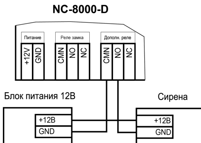
Рисунок 17. Схема подключения сирены к дополнительному реле
