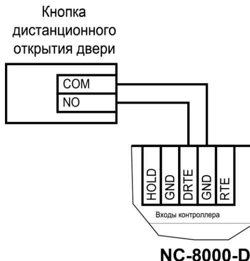
Рисунок 13. Схема подключения кнопки дистанционного открывания двери
