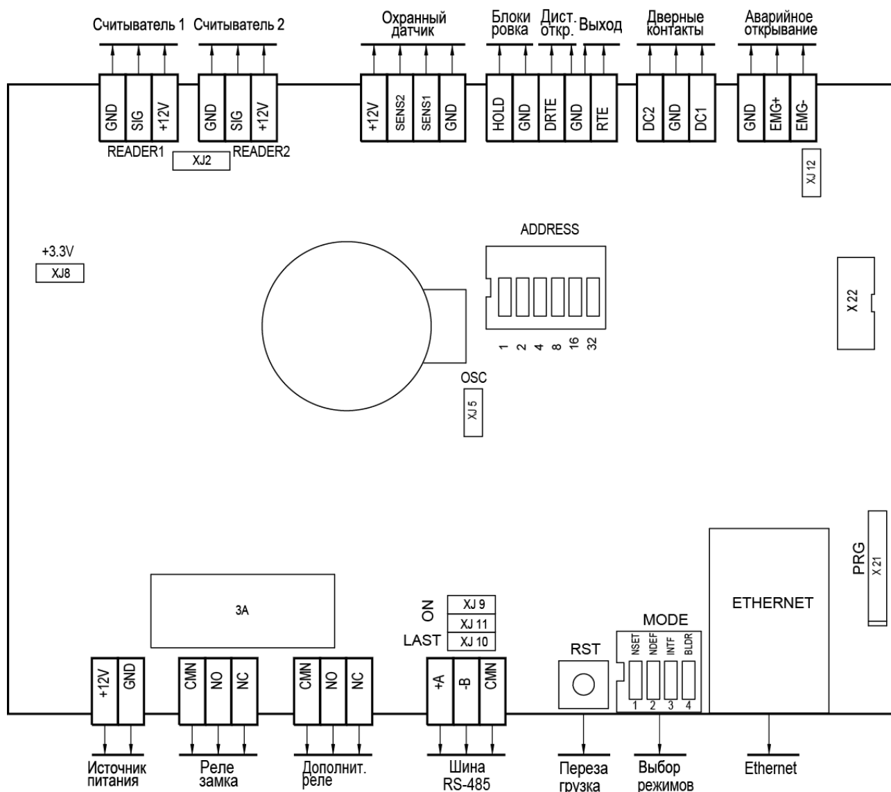
Рисунок 3. Схема платы контроллера NC-8000-D
