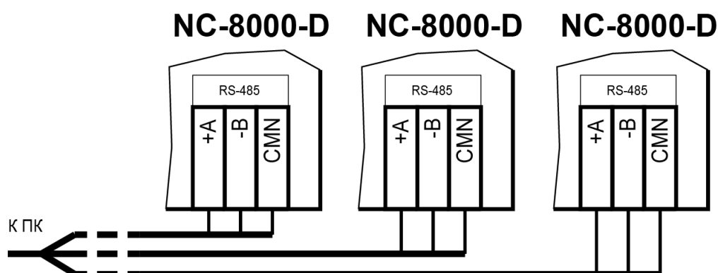
Рисунок 21. Пример соединения контроллеров по топологии «Звезда»
