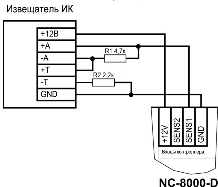
Рисунок 15. Схема подключения охранного датчика с контролем состояния линии
