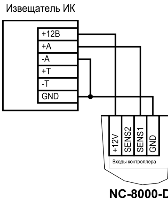
Рисунок 16. Схема подключения охранного датчика без контроля состояния линии
