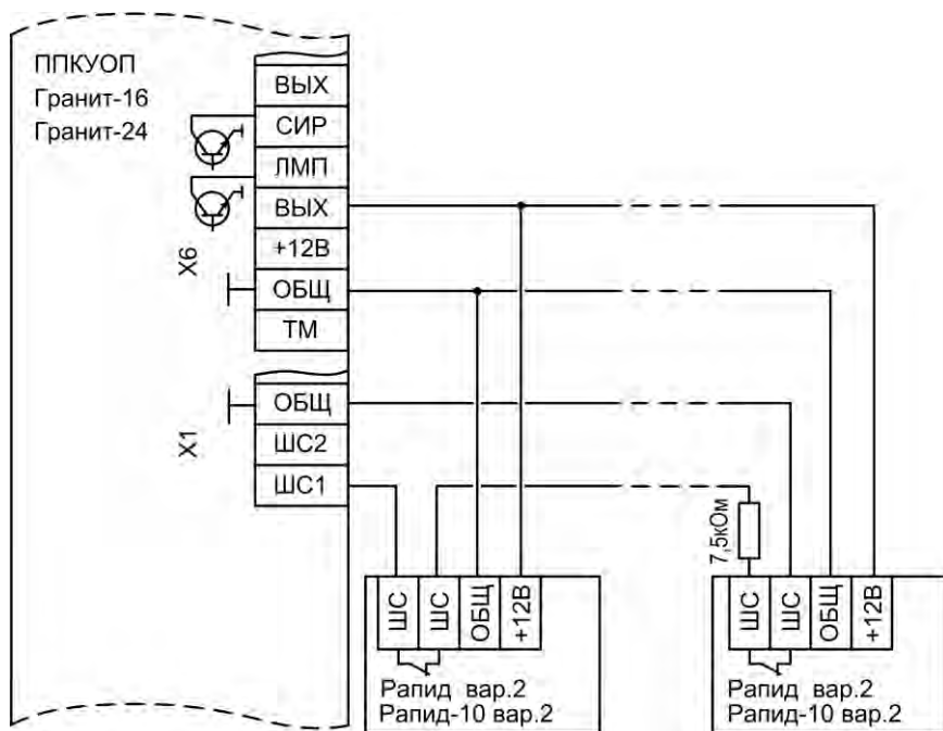
Рис.А5 Схема подключения охранных извещателей Рapid вар.2, Rapid-10 вар.2
