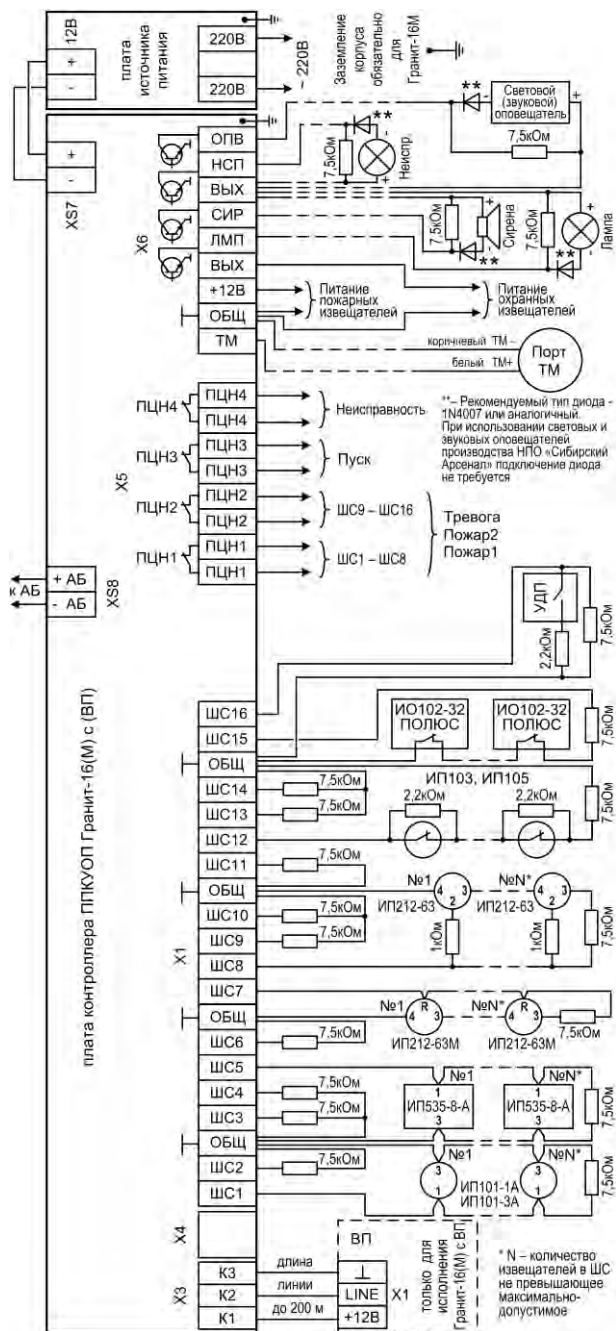
Рис.А1 Схема внешних подключений ППКУОП Гранит-16(М) с (ВП)
