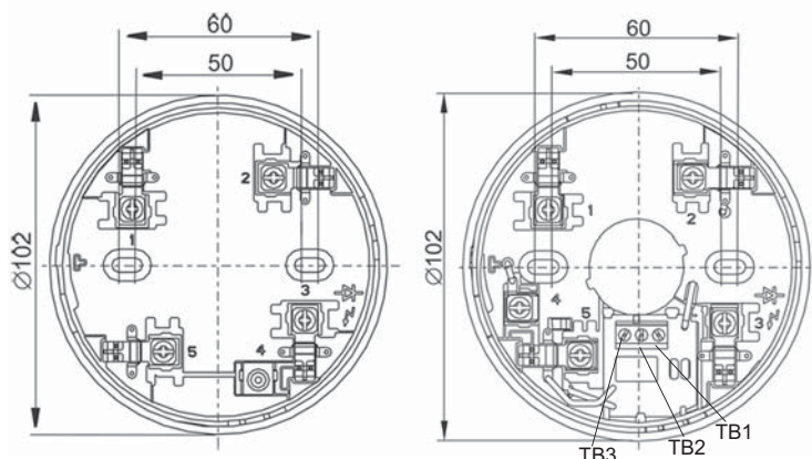
Базы E1000B, E1000R
