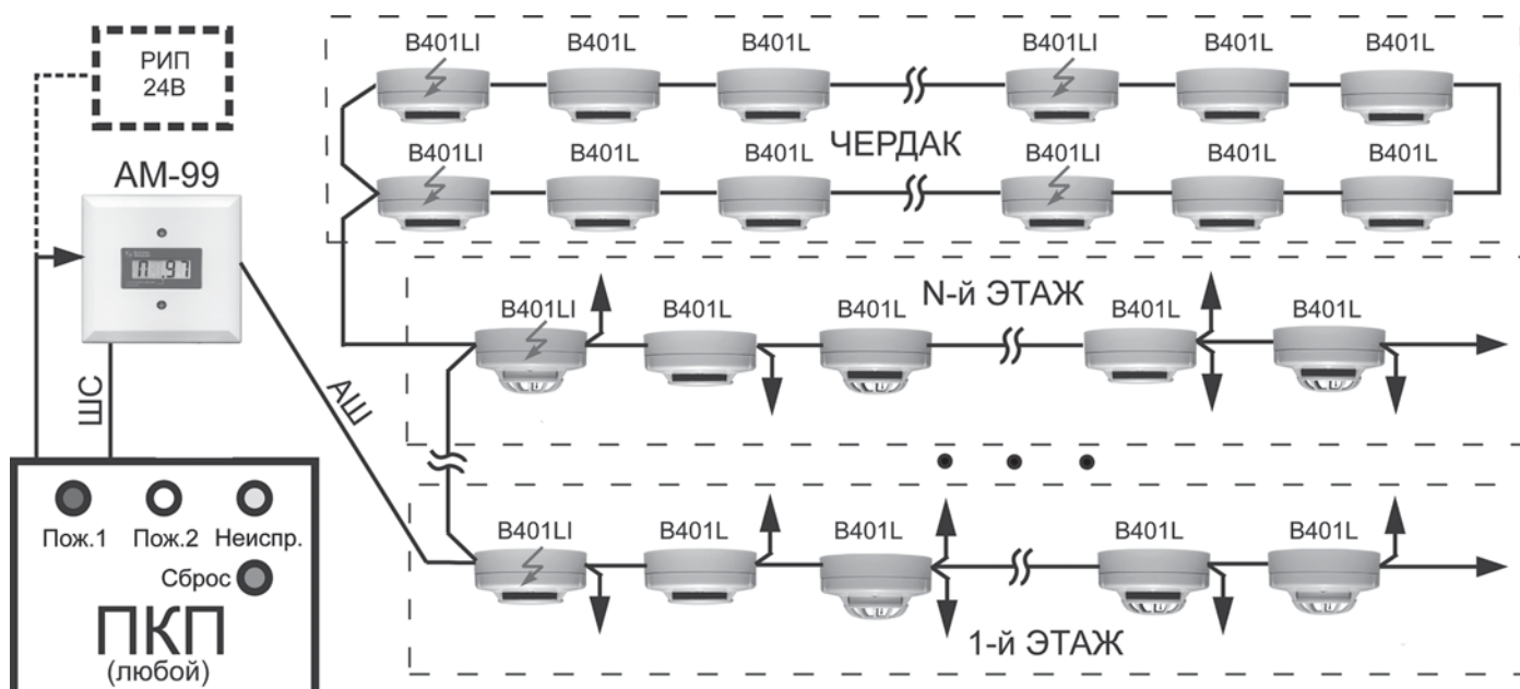
Вариант построения системы пожарной сигнализации, выполненной на базе серии Леонардо.
