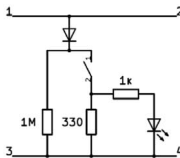
Эквивалентная схема
