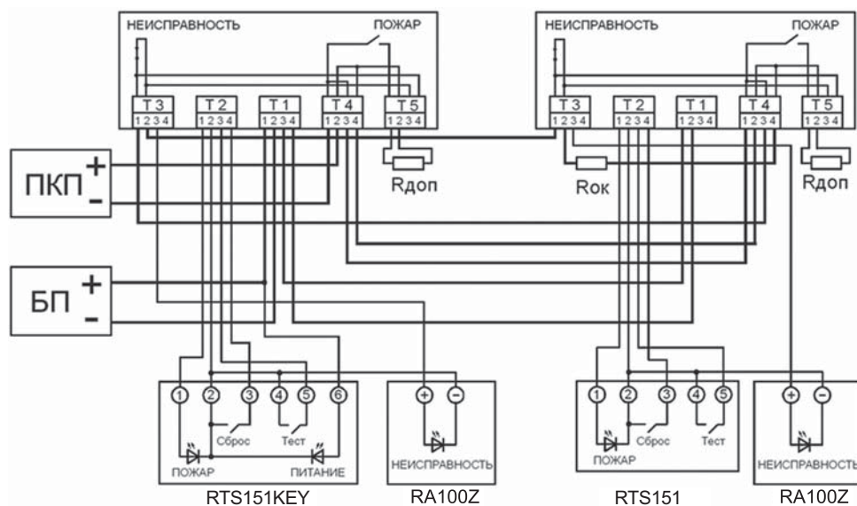
Схема подключения ПКП с постоянным напряжением в шлейфе
