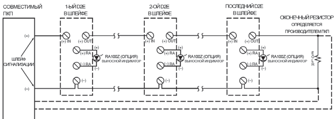
Схема подключения D2E в шлейф приемно-контрольного прибора (ПКП)
