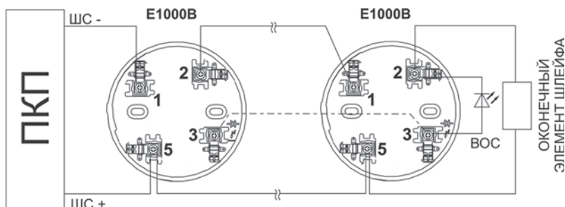
Схема подключения баз E1000B к однопороговому ПКП (без распознавания двух сработавших извещателей в шлейфе) с ограничением тока шлейфа до 80 мА
