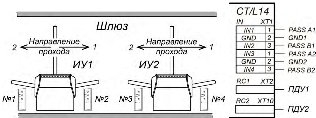
Рисунок 26. Схема шлюза из двух турникетов
