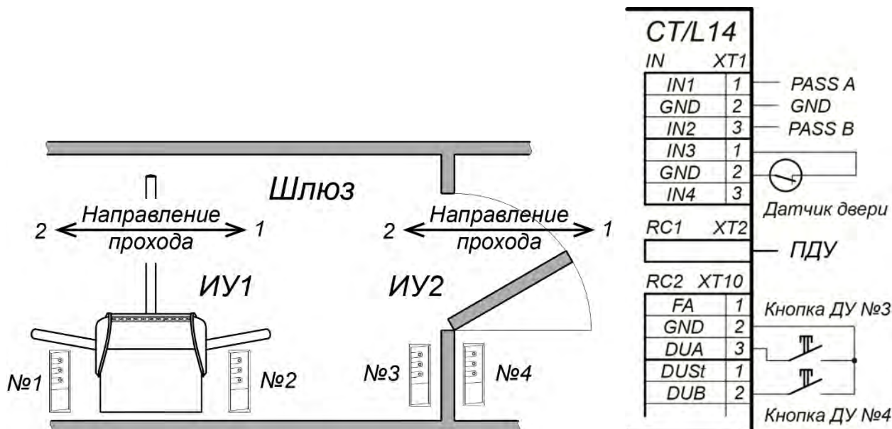
Рисунок 25. Схема шлюза из турникета и замка
