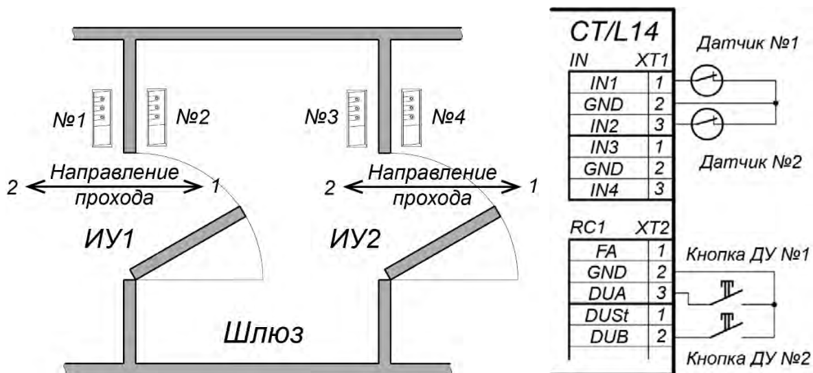
Рисунок 23. Схема шлюза из замков
