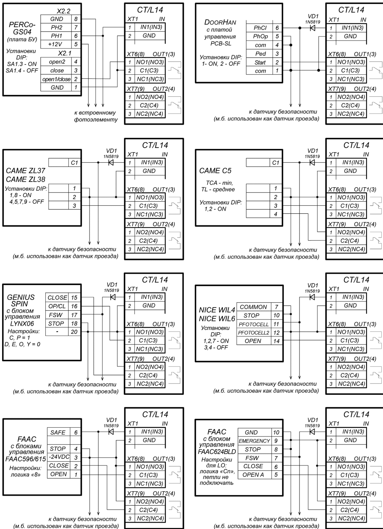
Рисунок 9. Примеры схем подключения шлагбаумов к контроллеру АТП
