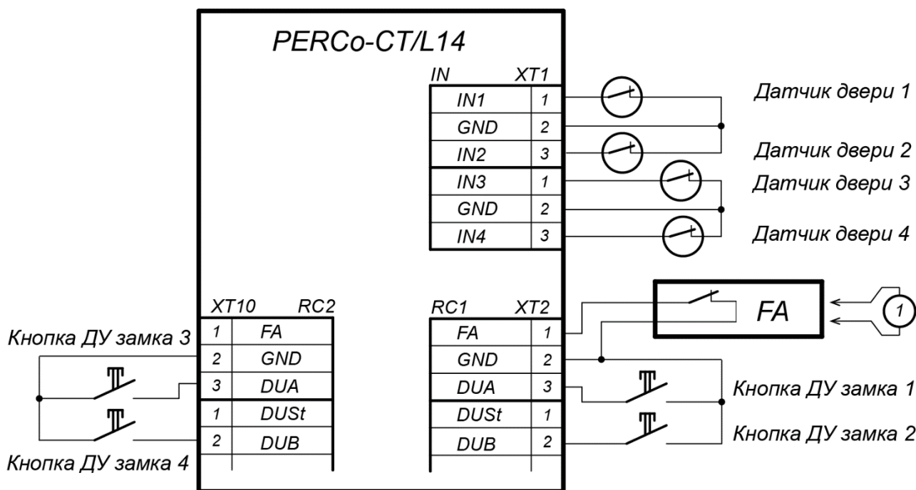
Рисунок 6. Схема подключений кнопок ДУ и датчиков двери
