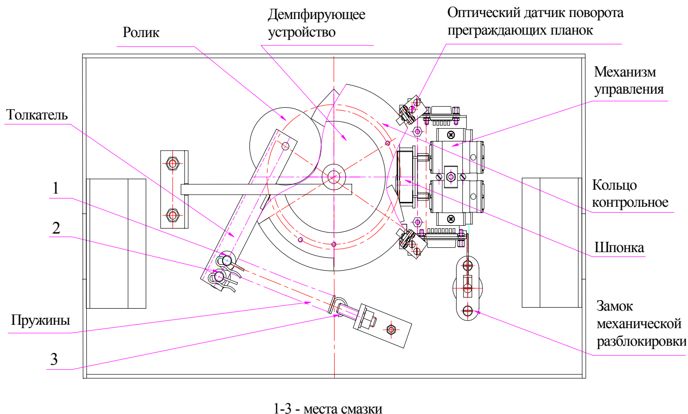
Рисунок 14 - Расположение внутренних деталей и узлов стойки турникета
