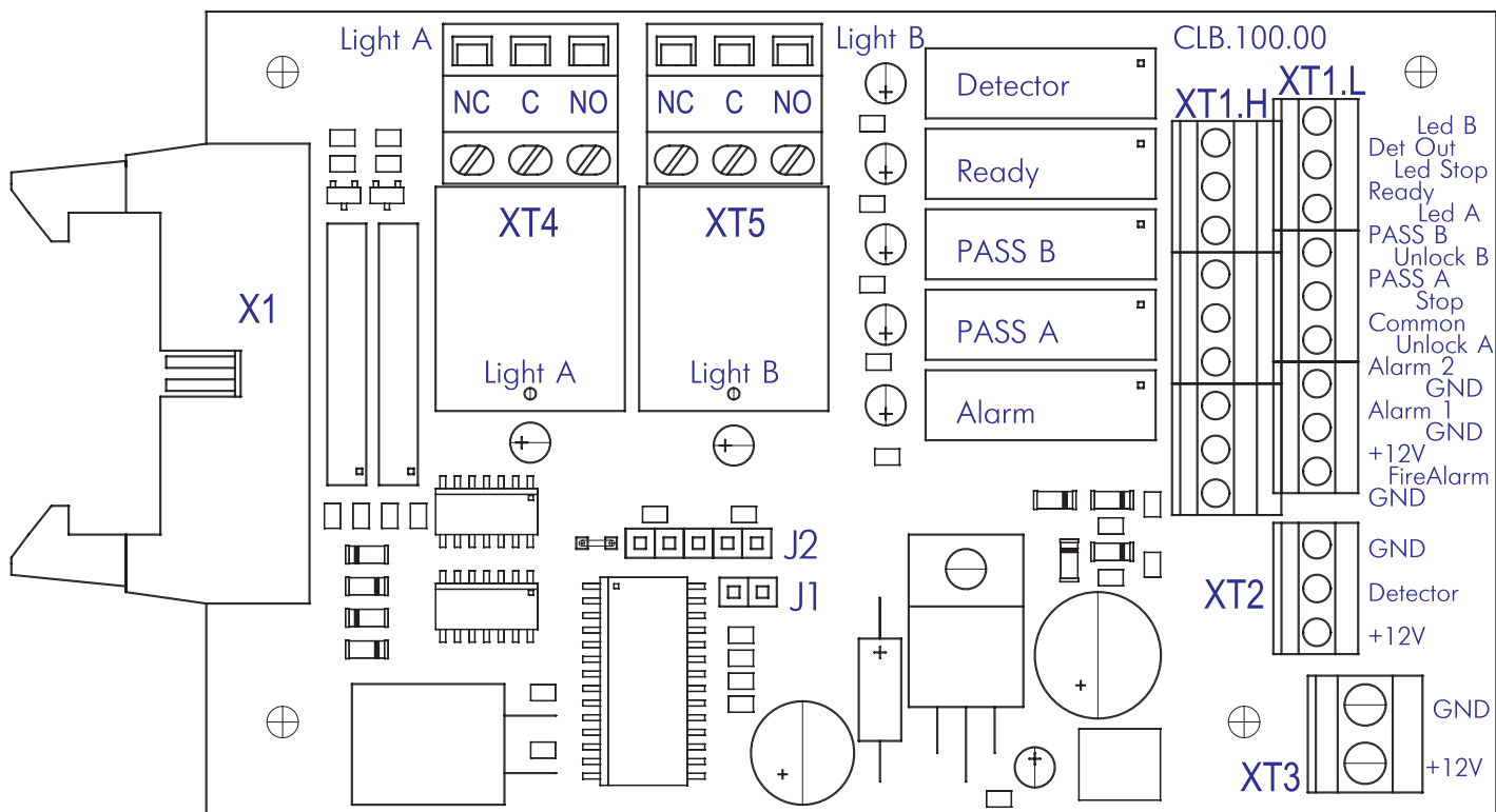
Рисунок 3 - Внешний вид платы CLB
