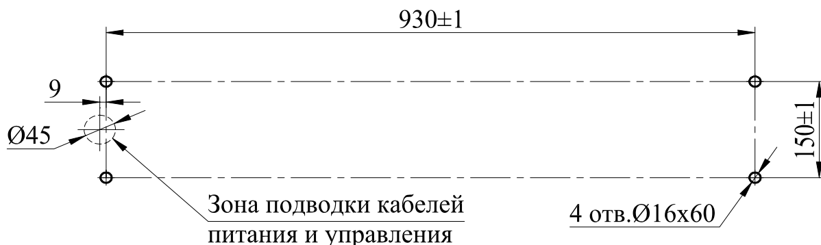
Рисунок 10 - Разметка отверстий для установки стойки турникета
