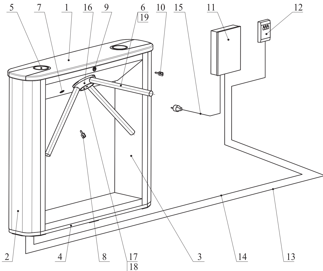
Рисунок 1 - Общий вид турникета
