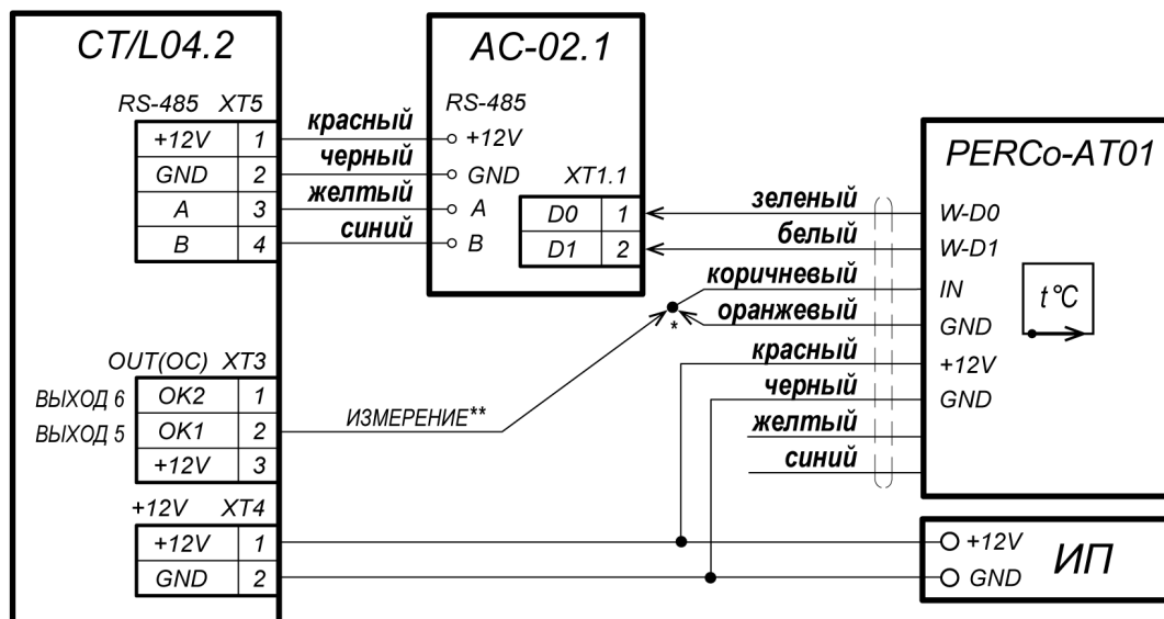
Рисунок 25. Схема подключения к контроллеру СТ/L04.2 пирометра PERCo-AT01 с конфигурацией «ВБУ с тактированием»
