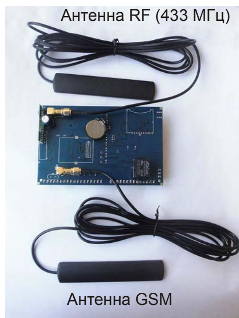
Антенна RF (433 МГц) Антенна GSM Внешняя антенна
