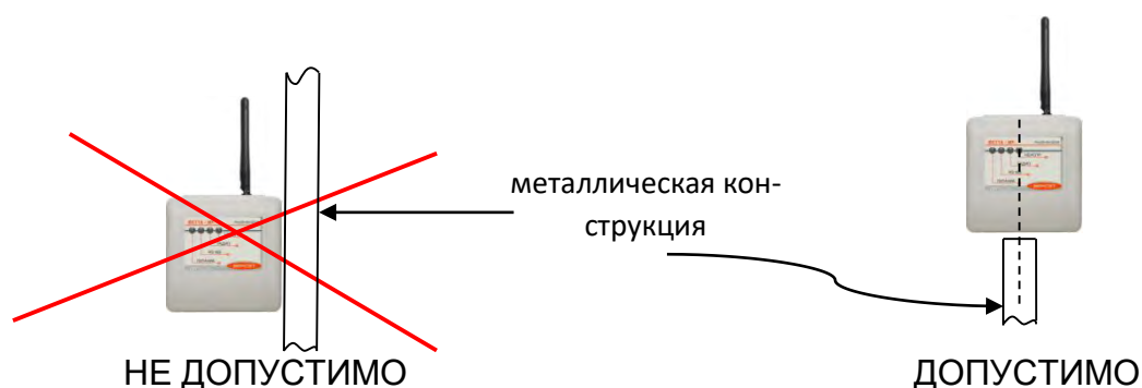
Рис. 2. Монтаж радиомодемов «ВЕТТА-MP» на металлическую мачту
