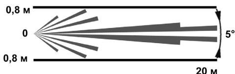
Рисунок 6 – Диаграмма зоны обнаружения извещателя ИО209-28 «Пирон-1А» (линейная зона обнаружения)
