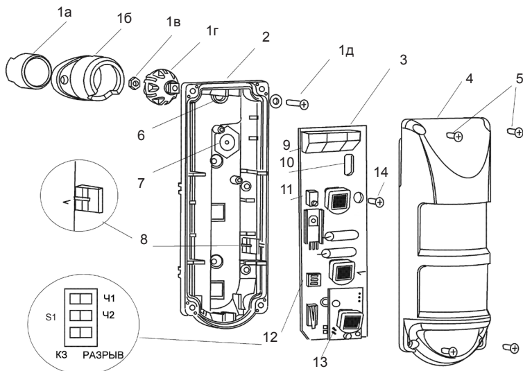
Рисунок 28 – Конструкция извещателя
