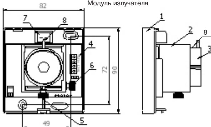
Модуль излучателя
