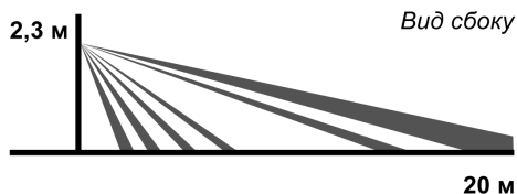
Вид сбоку
