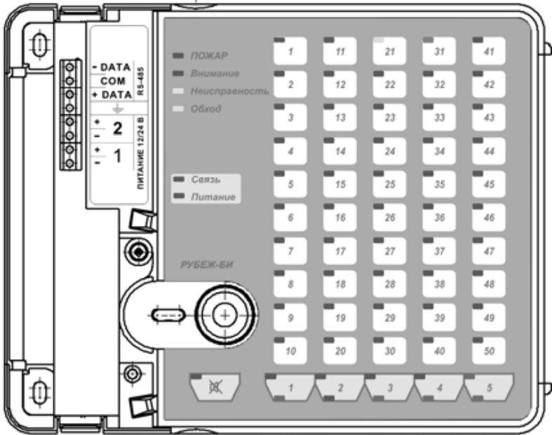
Рисунок 1 - Внешний вид прибора
